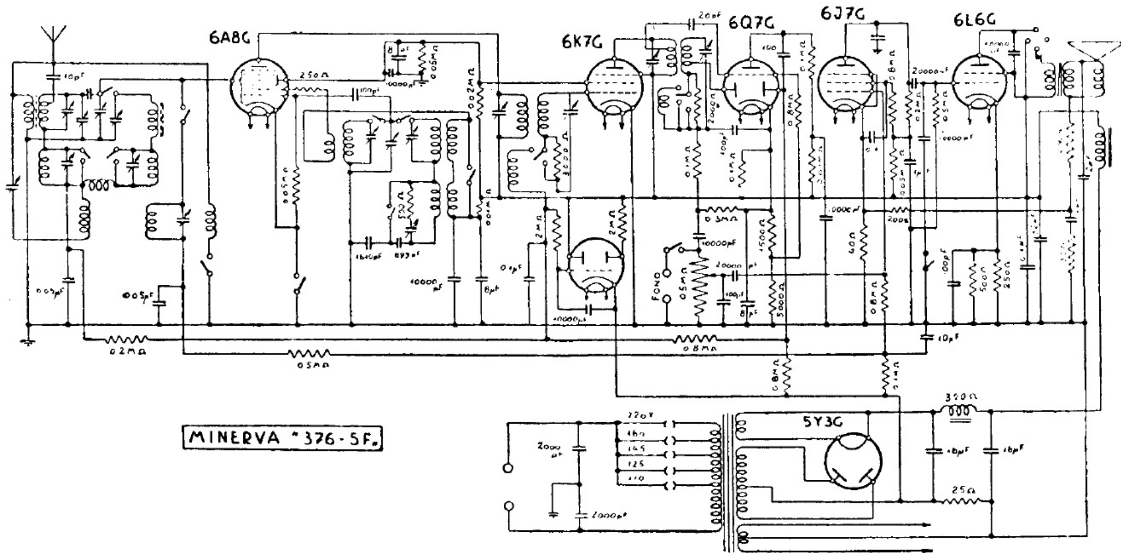
ITAL-MINERVA. — Mod. 376 SF. — Produzione 1938. — Media frequenza: 128 kHz. (La sezione triodo della 6Q7 amplifica il segnale prima della rivelazione per il c.a.v.).
